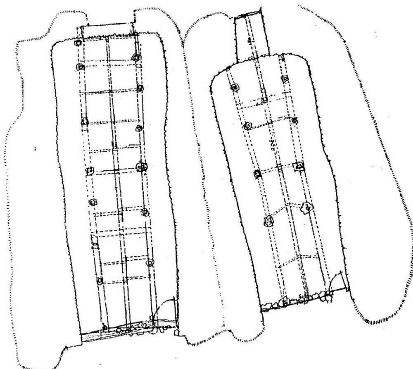
Hlöður í Selinu, grunnmynd. Teikning Curt von Jessen.
